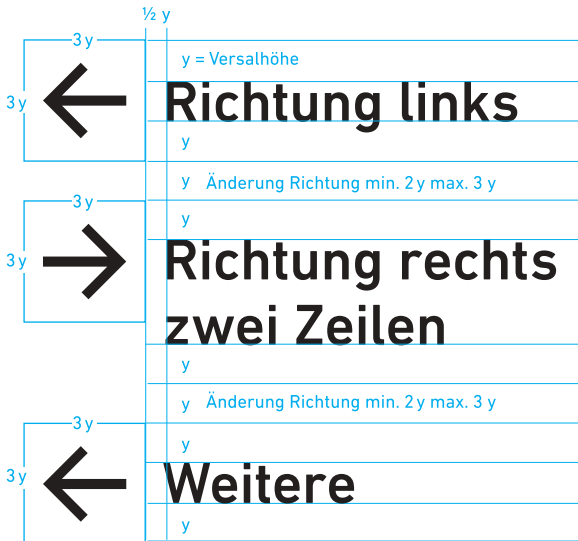
Allgemeine Definitionen Richtungspfeile
